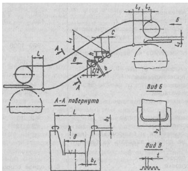
Схема устройства и основные размеры эскалатора
